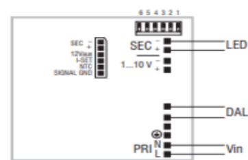
DALI diagram - Collegamento DALI
