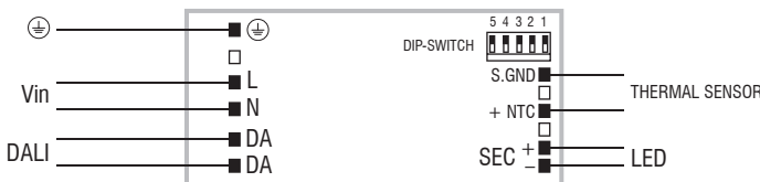
DALI diagram - Collegamento DALI
