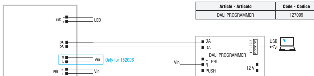
Programming via DALI - Programmazione tramite DALI
