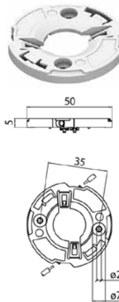
Holder 8201/G2
