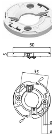
Holder 8201/G2
