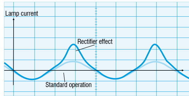
Fig. 7 - Rectifier effect
