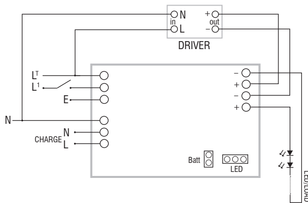
Maintained with external electronic driver diagram Collegamento permanente (illuminazione ordinaria)
