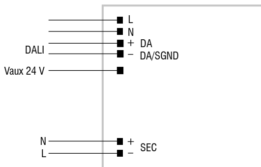
WIRELESS PROGRAMMING diagram Collegamento per PROGRAMMAZIONE WIRELESS
