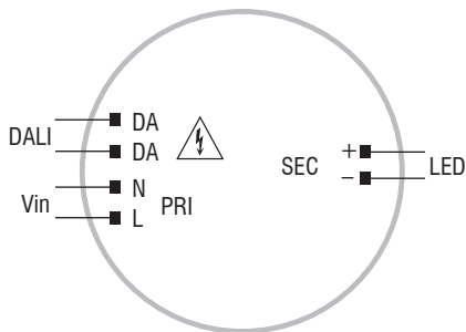
DALI diagram Collegamento DALI
