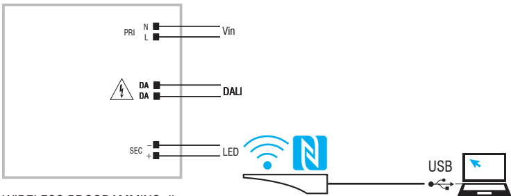
WIRELESS PROGRAMMING diagram Collegamento per PROGRAMMAZIONE WIRELESS
