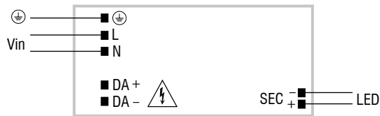
Active DALI diagram Collegamento DALI attivo
